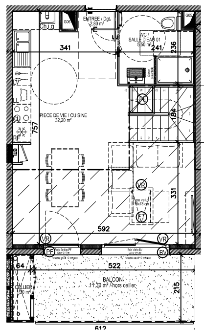
Plan R+1 (Niveau bas)
