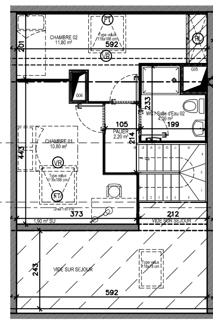
Plan R+C (Etage sous combles)
