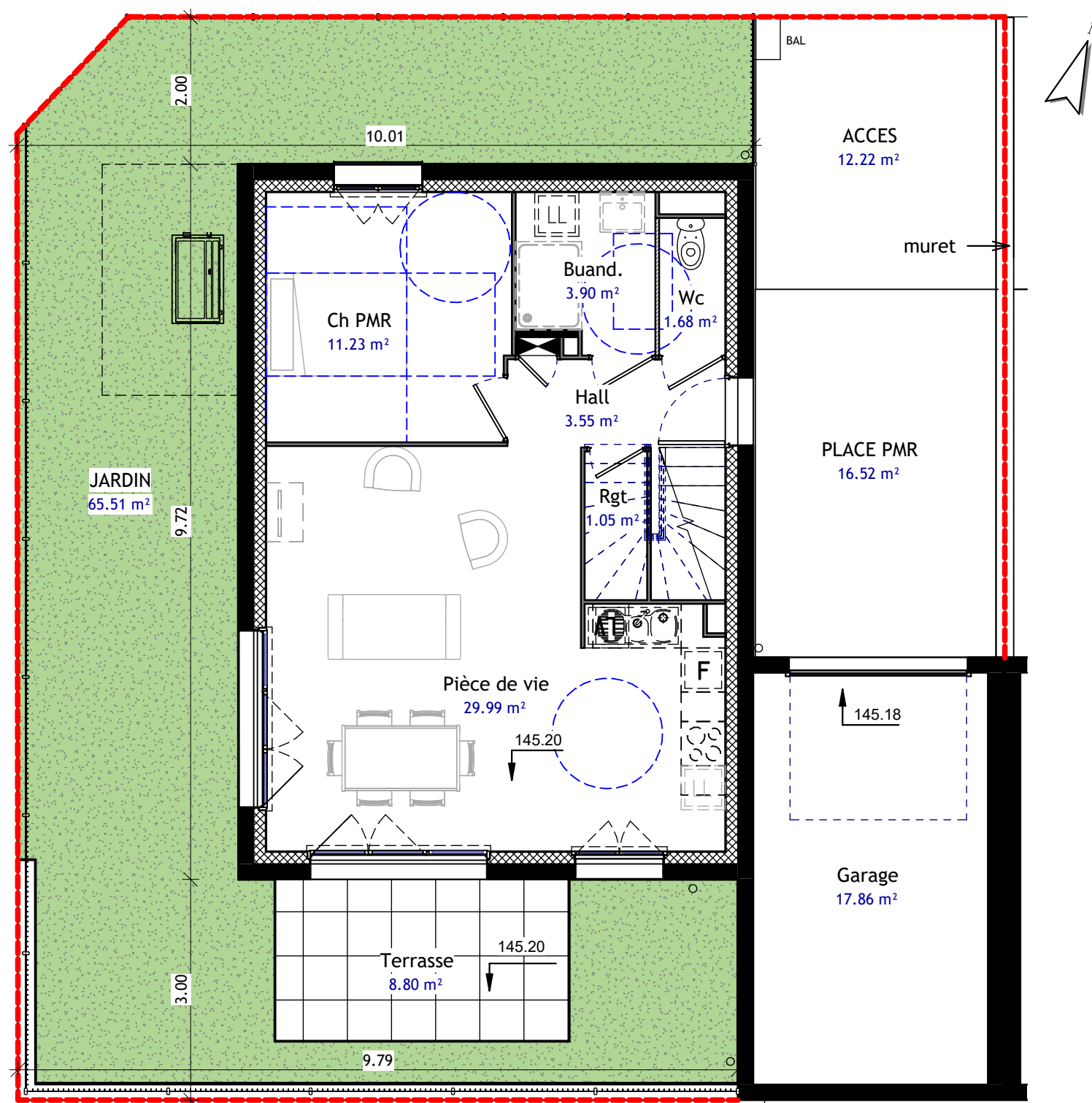
2 PDV VILLA 10 Ech : 1 : 75
